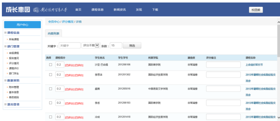
图 7.4.1 评分情况
