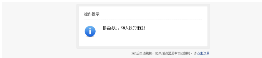
图 3.3.5 报名成功
