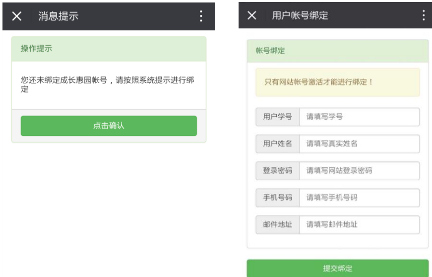
图 2.1.2 账号绑定
