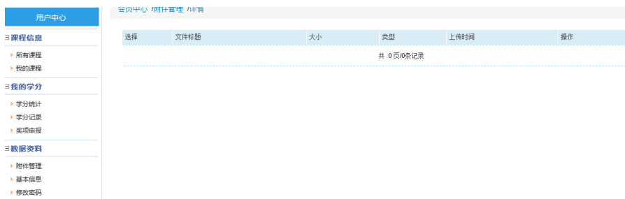
图 3.2.4 附件管理
