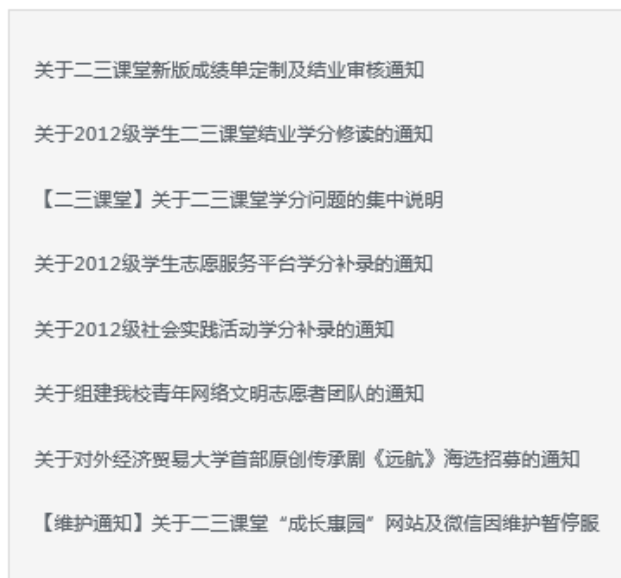
图 1.2 通知公告栏
