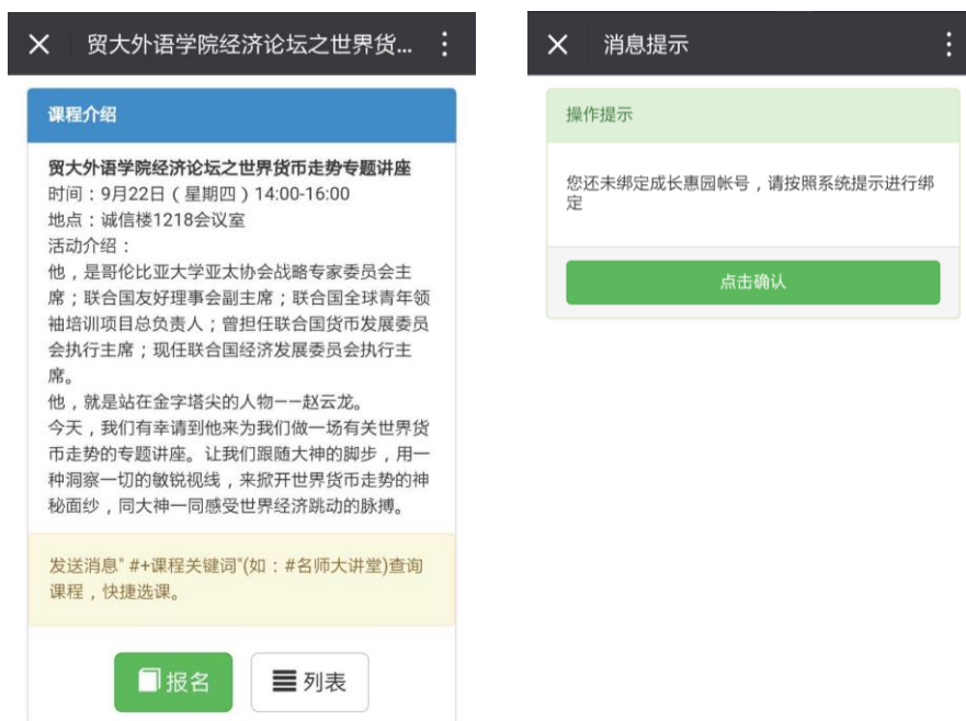
图 6.2 课程报名
