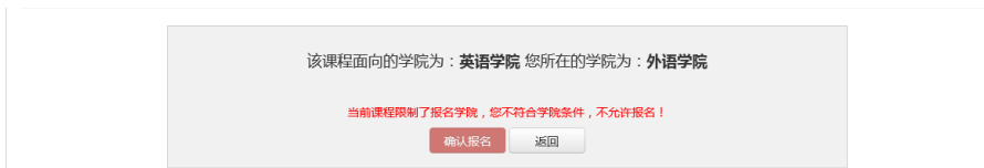
图 3.3.4 不符合条件
